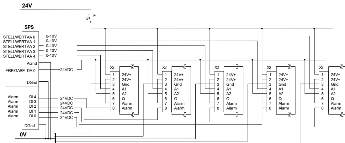
Abbildung 12 - Ausführung mit individueller Alarm-Auswertung
