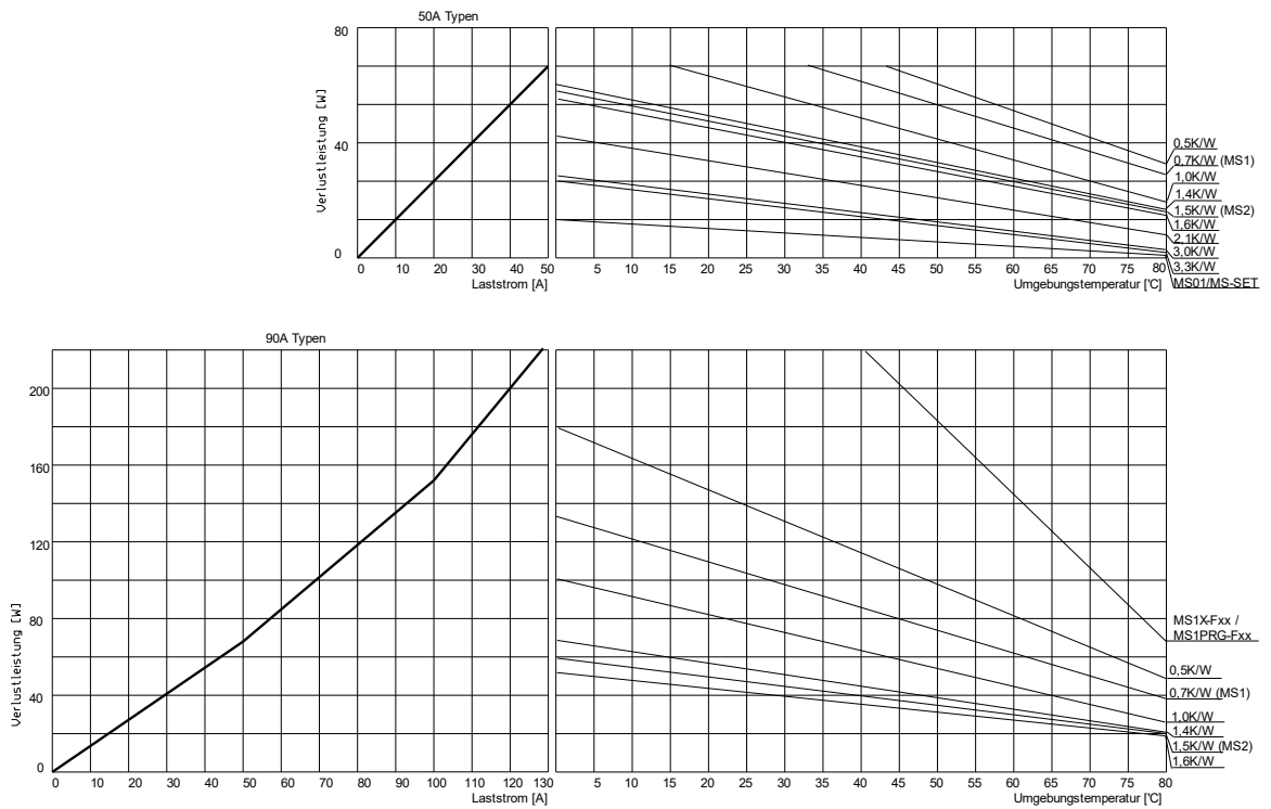
Abbildung 6 - Derating Kurven
