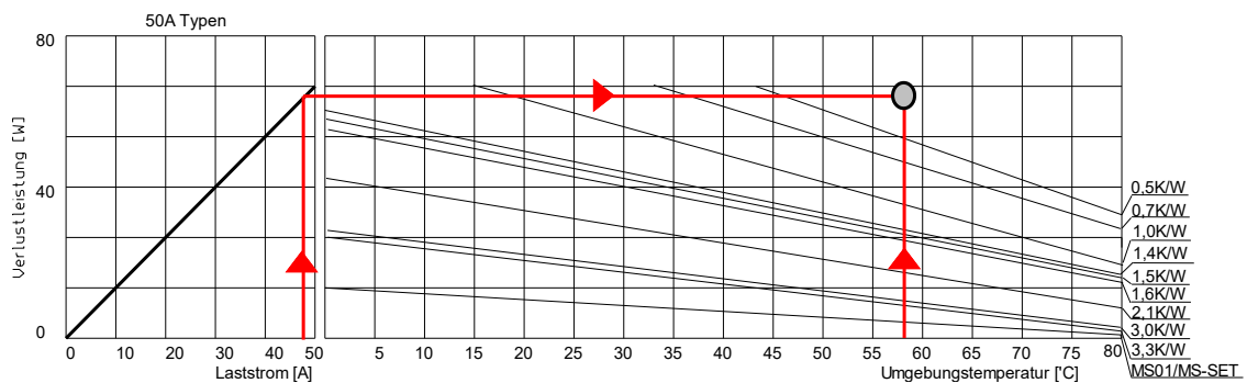
Abbildung 14 - Beispiel Kühlleistung PR4850
