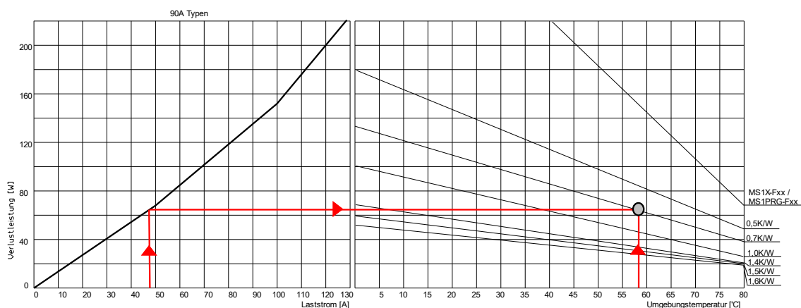
Abbildung 15 - Beispiel Kühlleistung PR4890
