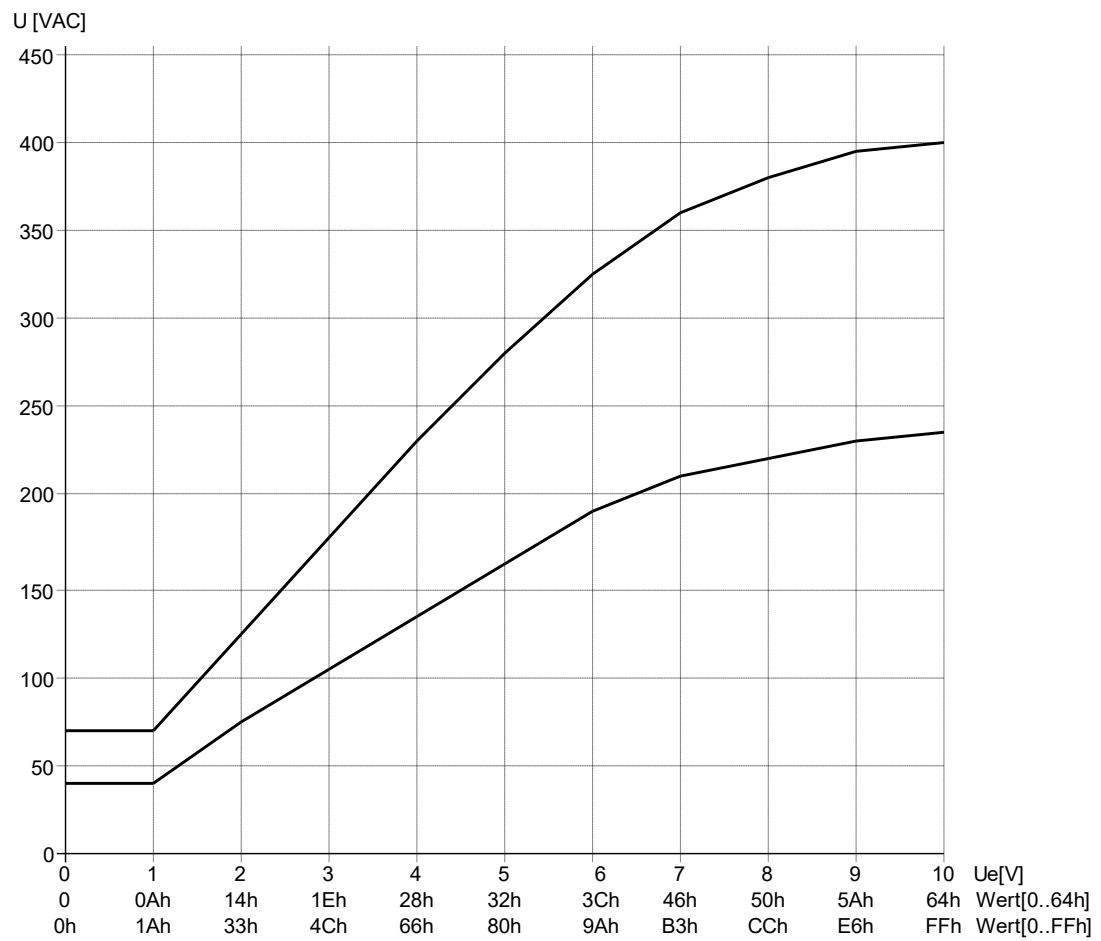
Abbildung 11 - Effektive Lastspannung via Steuerspannung
