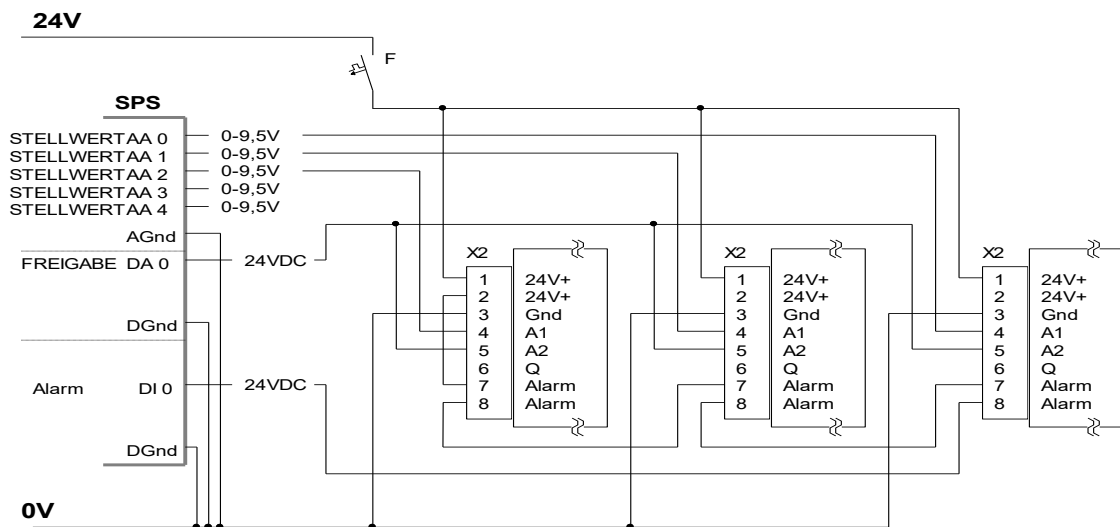
Abbildung 13 - Ausführung mit Summen-Alarm-Auswertung
