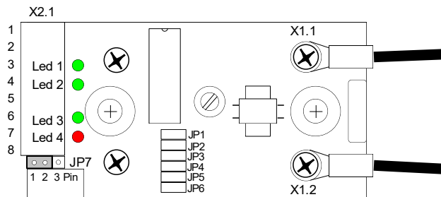
Abbildung 17 - Bedeutung der LEDs
