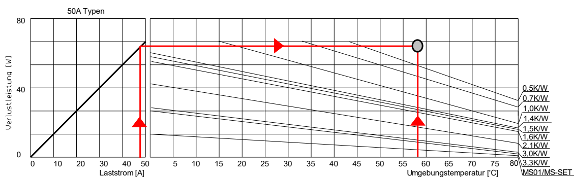
Abbildung 15 - Beispiel Kühlungsforderung PR4850
