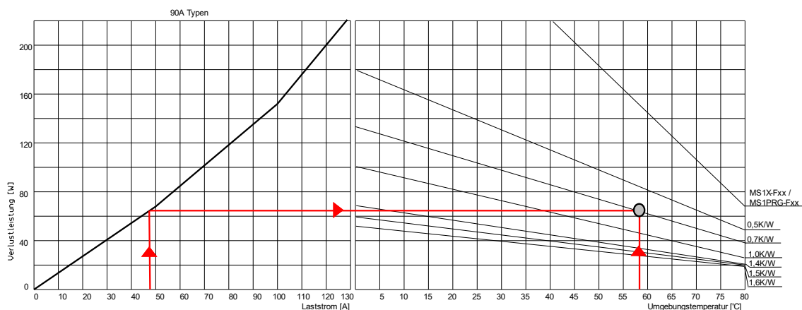
Abbildung 16 - Beispiel Kühlungsforderung PR4890
