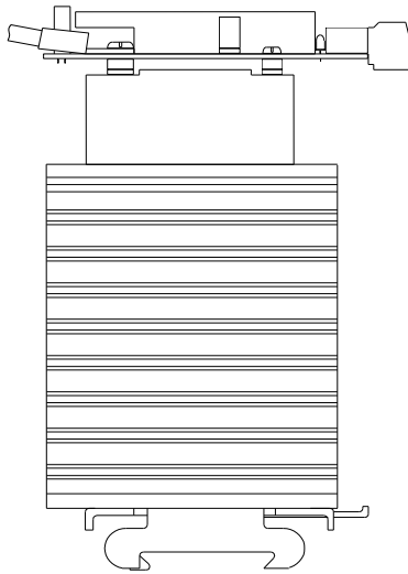
Abbildung 5 - Ausführungsbeispiel PR4890-3261
