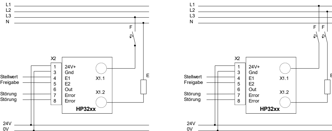
Abbildung 4 - typischer Anschluss 230V / 400V
