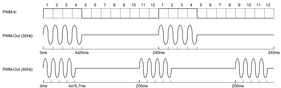
Abbildung 5 - Lastspannung als Funktion der Eingangs-PWM (Stellwert = 4) bei 50Hz bzw. 60Hz
