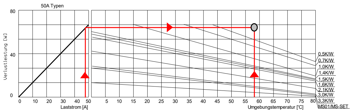
Abbildung 10 - Beispiel Kühlanforderung PR4850
