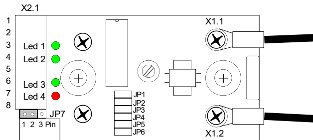
Abbildung 2 - Lage der Stecker, Jumper und LEDs
