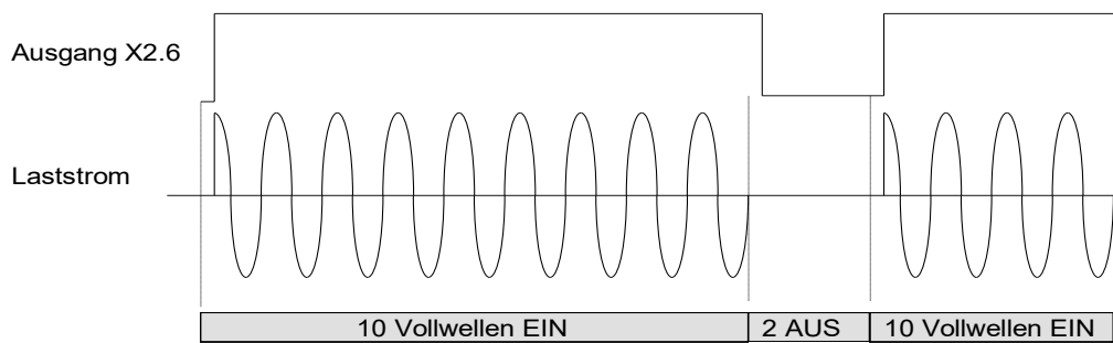
Abbildung 7 - Darstellung der Lastspannung bei Stellwert = 10 und Jumper 1 gesteckt, darüber der Verlauf der Spannung an Klemme X2.6
