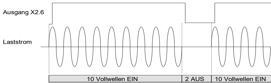
Abbildung 6 - Darstellung der Lastspannung bei Stellwert = 10, darüber der Verlauf der Spannung an Klemme X2.6
